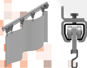
Detalle carros maestros y de seguimiento
