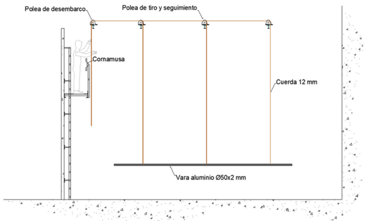
Esquema funcionamiento TMN
